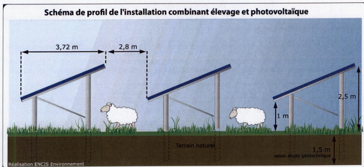
Schéma de profil de l'installation prévue combinant élevage et photovoltaïque Source : ENCIS Environnement
